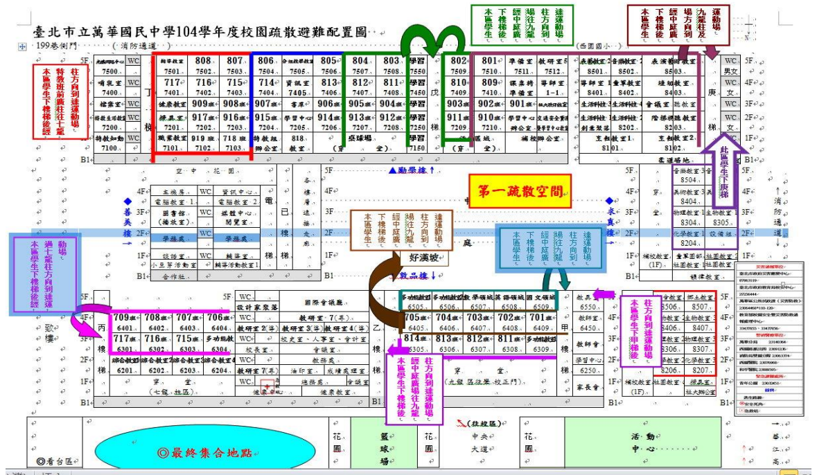
圖 8-2-3、避難逃生校舍全景路線圖
